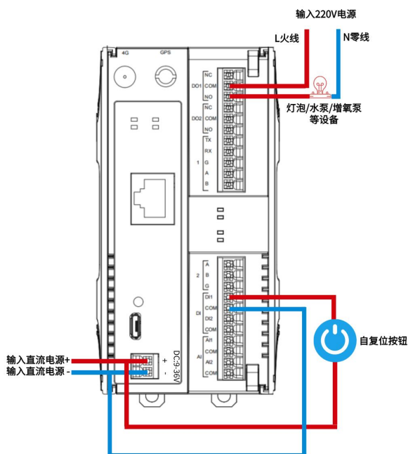
(1) 【手动控制开关接线图】
