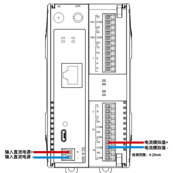
(3) 【采集电流值接线图】
